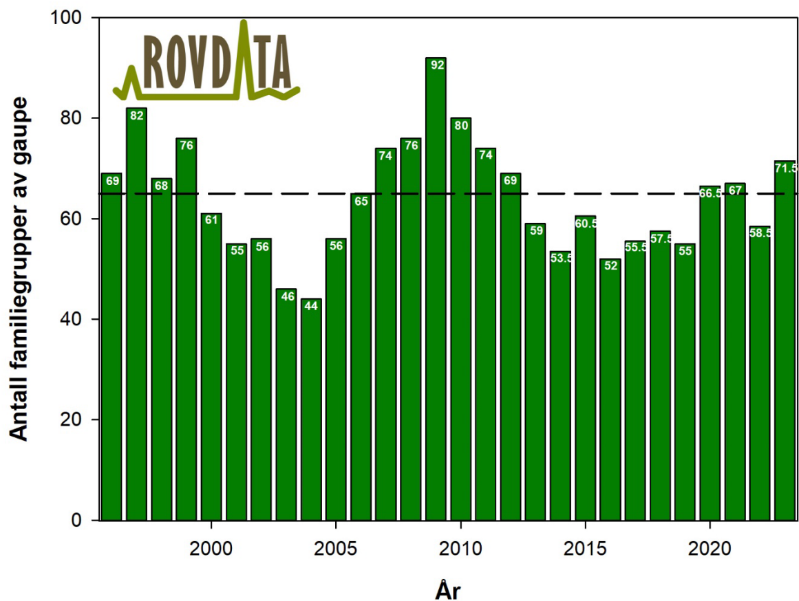
Figur 4. Antall familiegrupper av gaupe på landsbasis før jakt i perioden 1996–2023. Den stippledde linjen angir det nasjonale bestandsmålet på 65 familiegrupper. Antall familiegrupper i 2014 og senere år er ikke direkte sammenlignbart med tidligere år, da overvåkingsmetodikken er endret i forbindelse med samordningen med Sverige.
