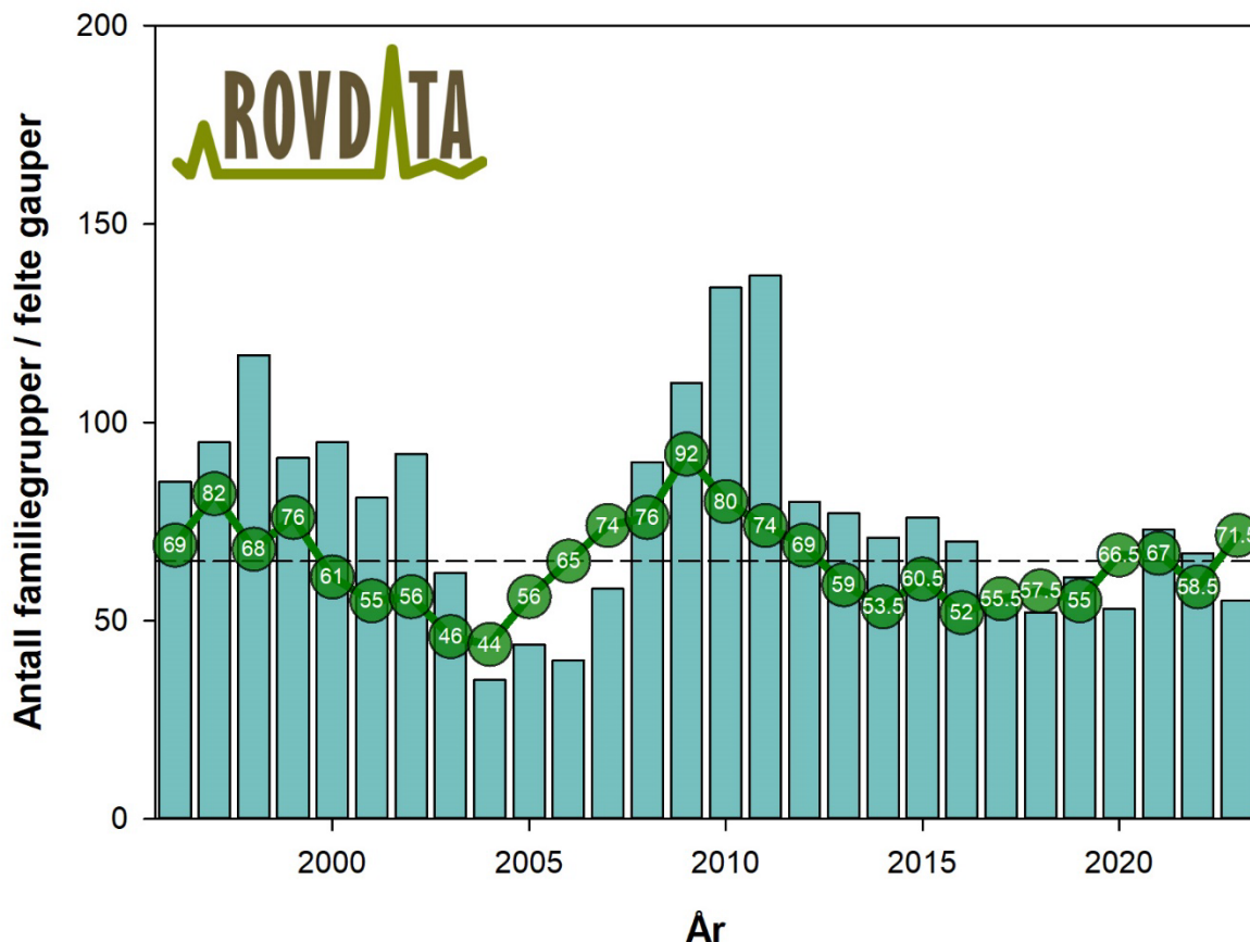
Figur 7. Antall familiegupper av gaupe (sirkler) og uttak av gauper (stolpediagram) i Norge i perioden 1996–2023. Antall familiegupper i 2014 og senere år er ikke direkte sammenlignbart med tidligere år, da overvåkingsmetodikken er endret i forbindelse med samordningen med Sverige.
