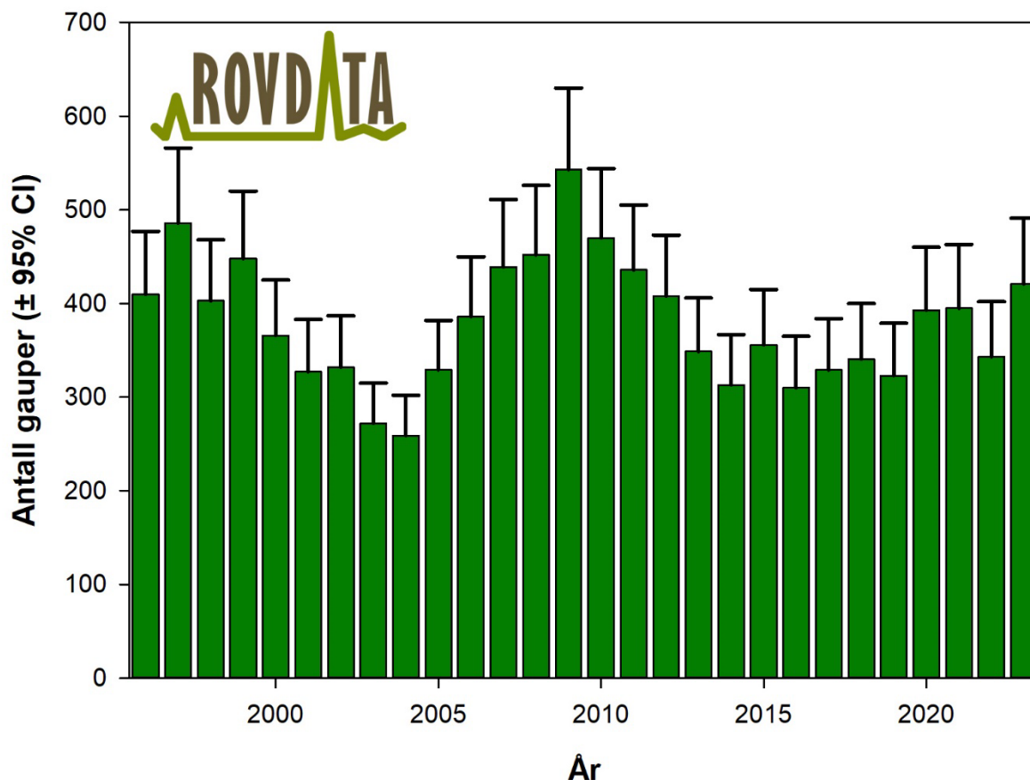
Figur 5. Estimert bestandsstørrelse (med 95 % CI) av gaupe på landsbasis før jakt i perioden 1996–2023. Bestandsestimatet for 2014 og senere år er ikke direkte sammenlignbart med tidligere år, da overvåkingsmetodikken er endret i forbindelse med samordningen med Sverige.
