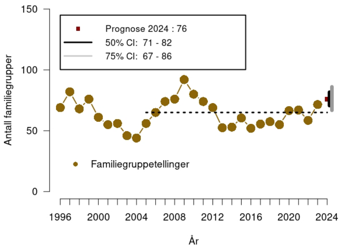
Figur 8. Utviklingen i gaupebestanden i perioden fra 1996 til 2023, samt modellprognoser for 2024 basert på informasjonen som er tilgjengelig i etterkant av jakta i 2023. Den stiplede linjen angir det nasjonale bestandsmålet på 65 familiegrupper.
