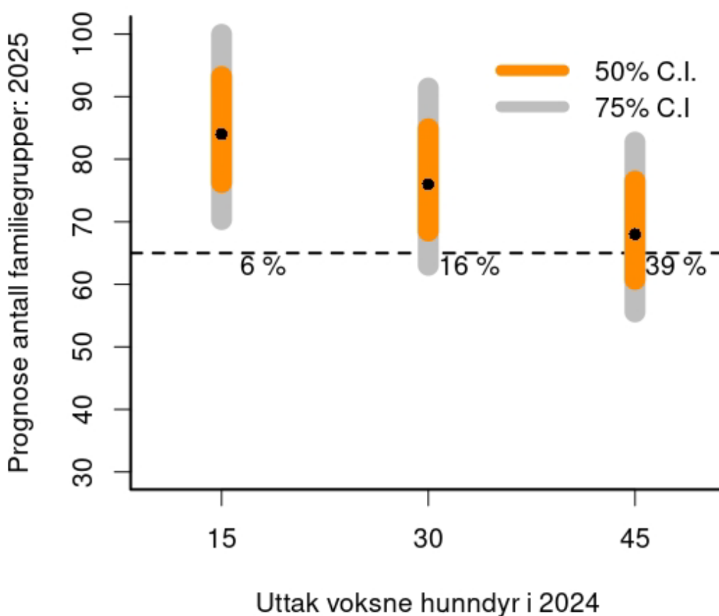
Figur 9. Prognose for antall familiegrupper på landsbasis før jakta i 2025 gitt tre ulike senarioer for uttak av voksne hunndyr under jakta i 2024 (henholdsvis 15, 30 og 45 voksne hunndyr). Sannsynligheten for å falle under bestandsmålet på 65 familiegrupper er hhv 6 %, 16 % og 39 % for de tre senarioene. Punkttestimatene (sort prikk) er hhv 84, 76 og 68 familiegrupper. Oransje strek angir 50 % CI og grå strek angir 75 % CI. Stiplet horisontal linje angir bestandsmålet på 65 familiegrupper.
